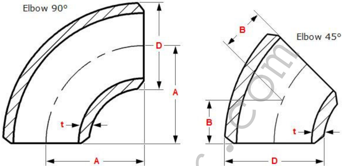
DIN 86090 - Butt Welding Fittings connecting with DIN 86019
