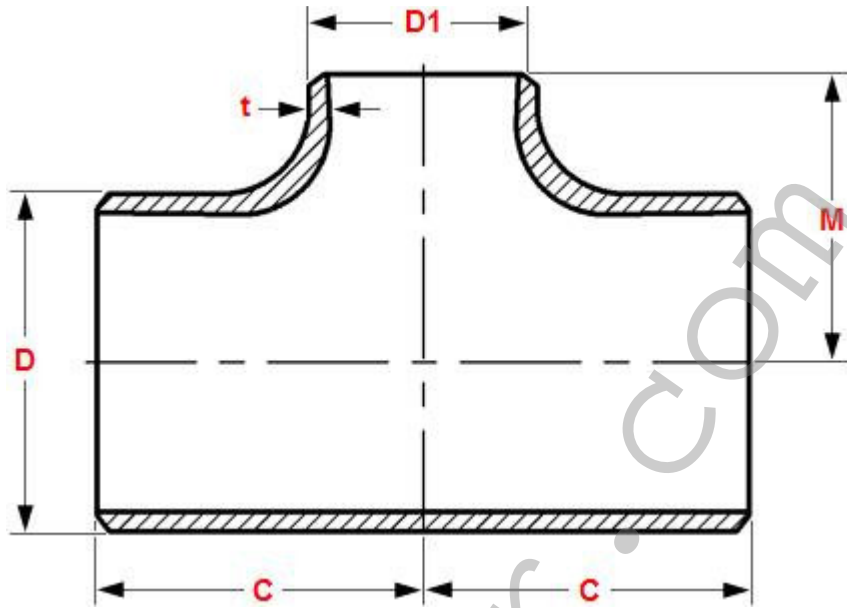
DIN 86088 - Butt Welding Fittings connecting with DIN 86019
